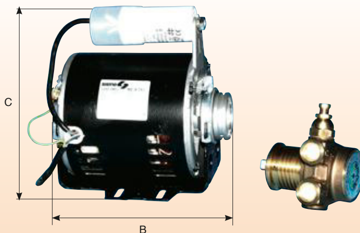
Motore monofase 4 POLI - 1 velocita' / 4 POLES - 1 speed single-phase motor
